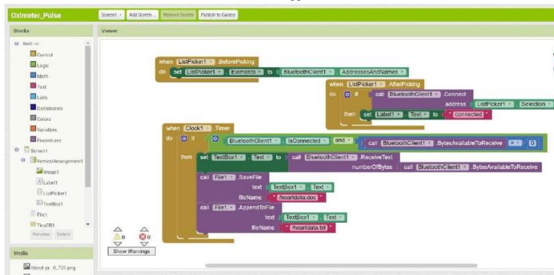
Figure 6 MIT App Inventor
